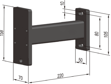
导轨水平支架
