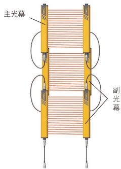
采用了补偿安装的串联设置
