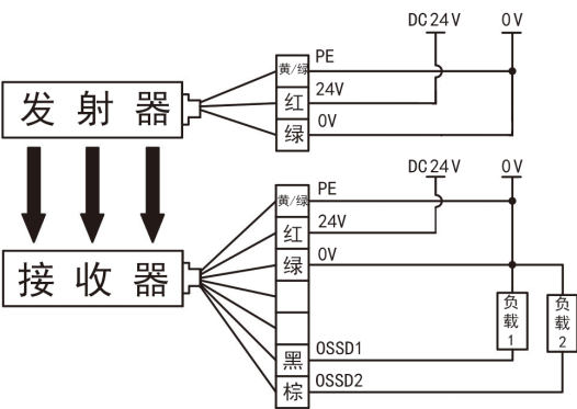
G 型，光同步编码 1 接线图
