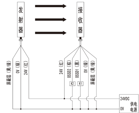
PNP, 光同步, 光通信编码 1
