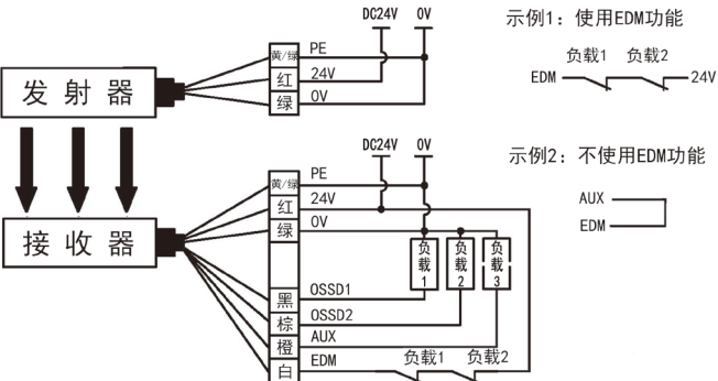
M 型，光同步编码 1 接线图
