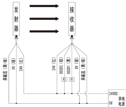
NPN，光同步，光通信编码 1
