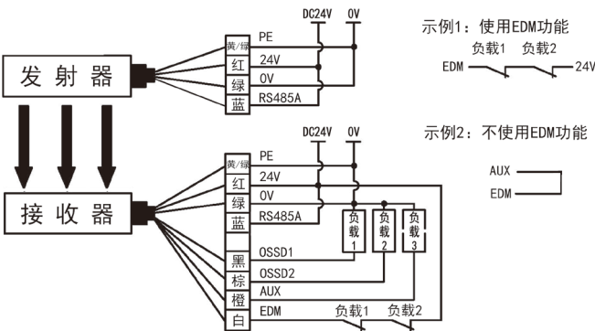
M 型，光同步编码 2 接线图
