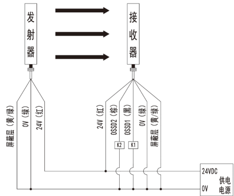
PNP，光同步，光通信编码 1
