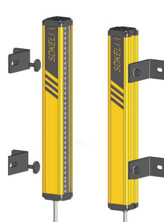
T 型槽安装方式 (TC)
