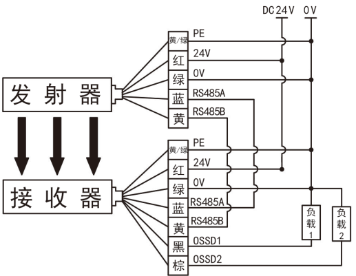
G 型，线同步接线图
