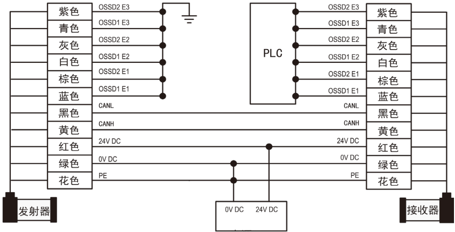
C型传感器单独接线图
