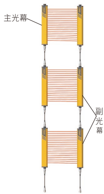
直接串联光幕间留有空隙
