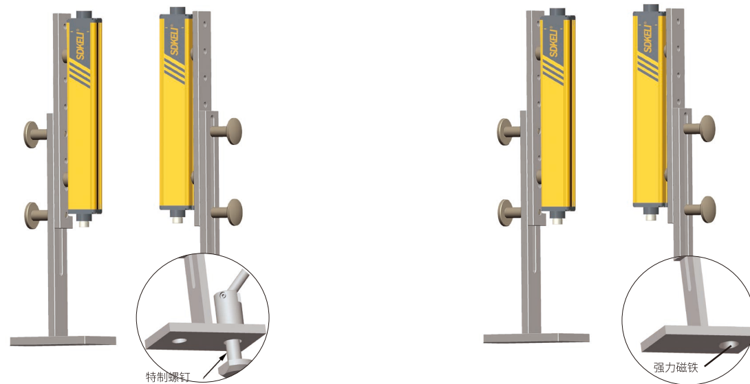
板状支架螺钉安装方式 (BL)
