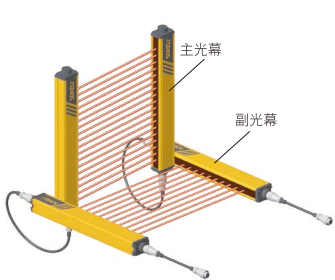
L 型设置时用到的补偿安装
