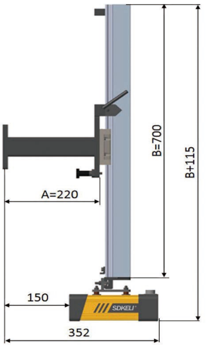
D型传感器导轨水平支架安装方式 (D7)
