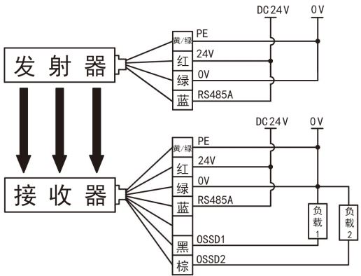
G 型，光同步编码 2 接线图
