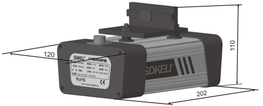
D型传感器外形尺寸
