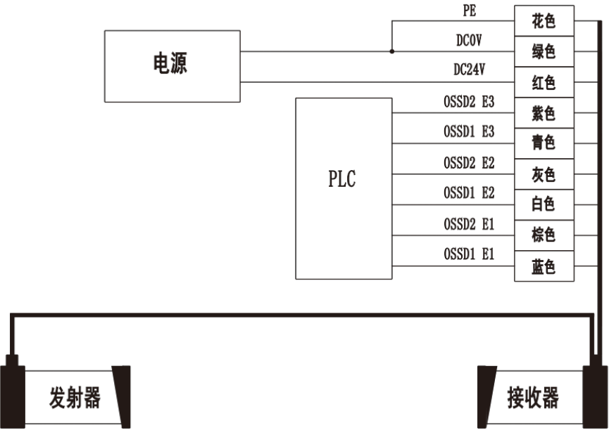
D型传感器单独接线图
