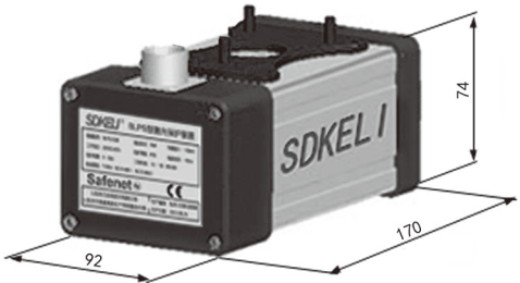
C型传感器外形尺寸
