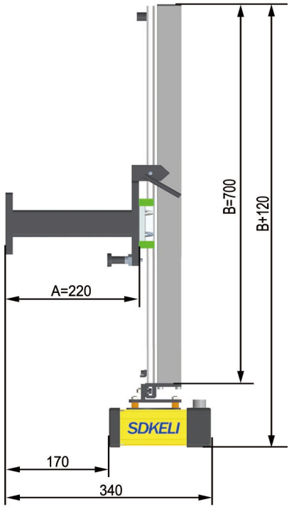
C型传感器导轨水平支架安装方式 (D7)
