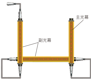
U 型设置时用到的补偿安装
